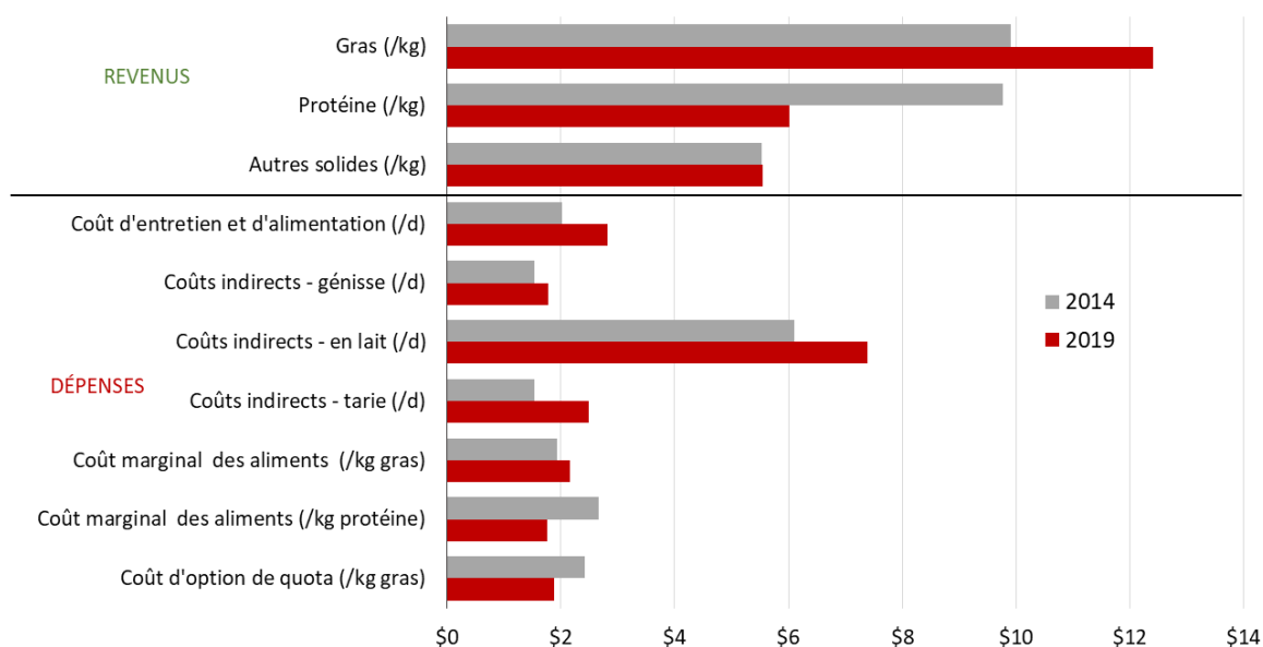
Figure 1 : Changement des valeurs économiques utilisées dans le calcul de la rentabilité des vaches Holstein
