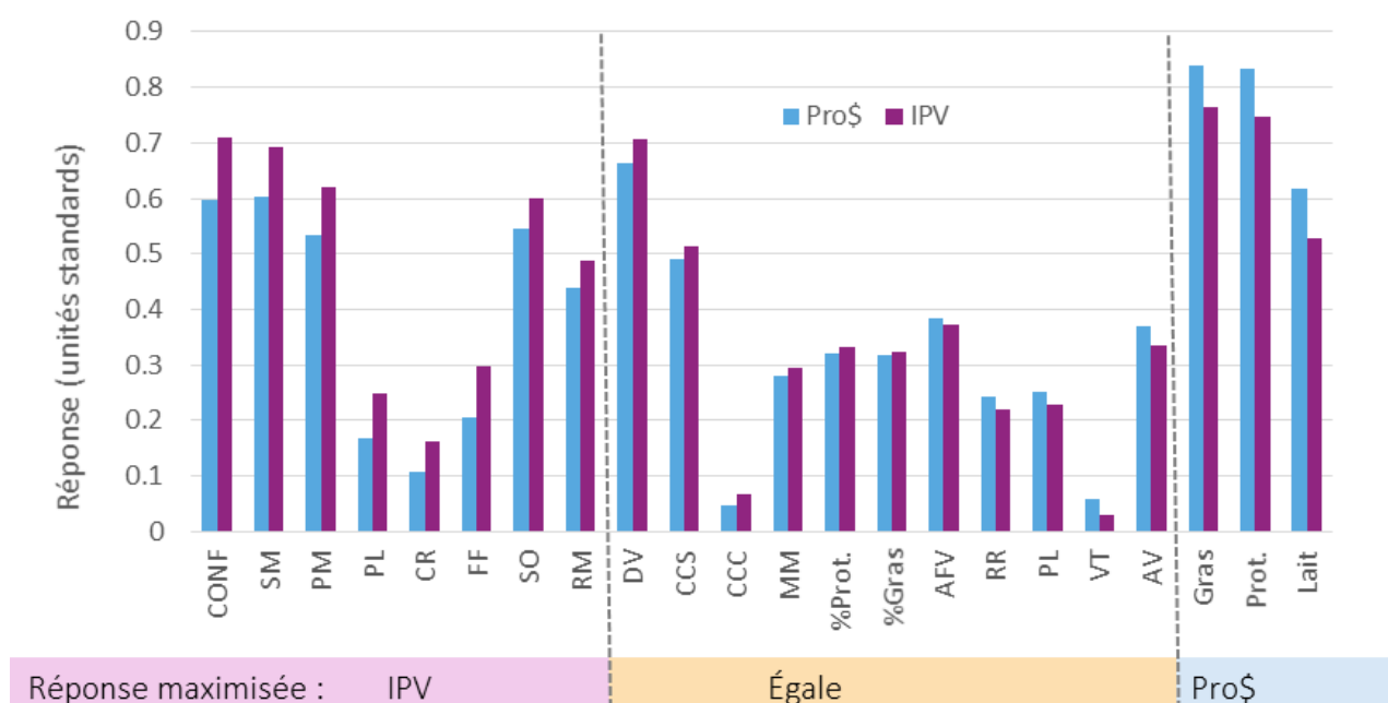
Figure 3 : Réponse prévue par caractère pour l'IPV et Pro$
